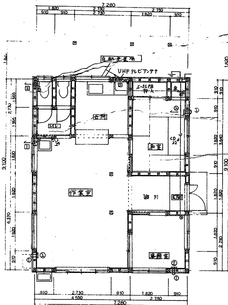
換気電話機TV平面図 1/50
