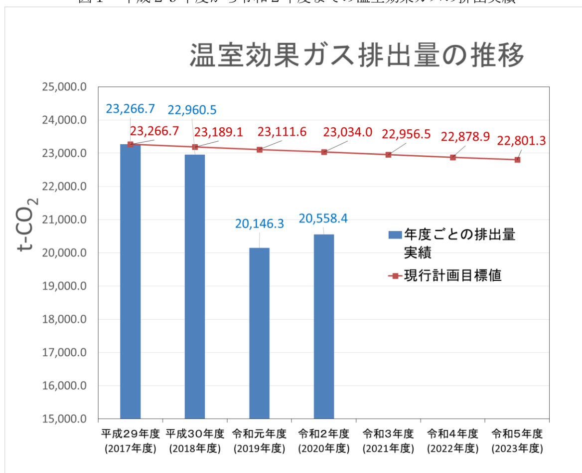
図1 平成29年度から令和2年度までの温室効果ガスの排出実績
