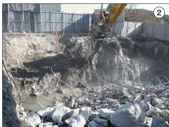
煙突の基礎部分の解体状況
