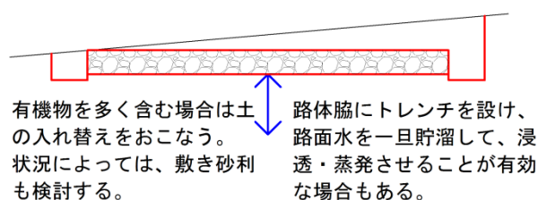
緩傾斜地における横断面形の一例
