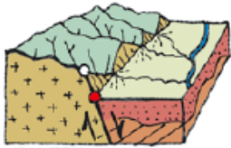
縦ずれ断層
