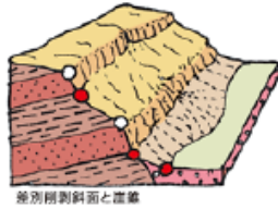
差別傾斜面と崖錐
