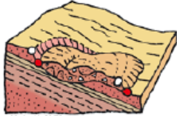
地すべり地形
