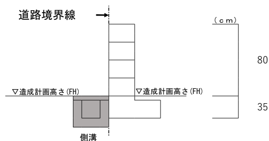
図2、施工済み道路境界の場合（ブロック設置の断面参考図）
