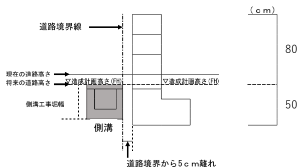
図3、道路未施工の場合（ブロック設置の断面参考図）
