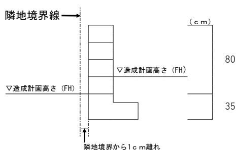
図1、隣地境界の場合（ブロック設置の断面参考図）
