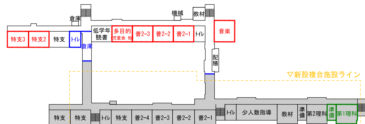
2階平面図
