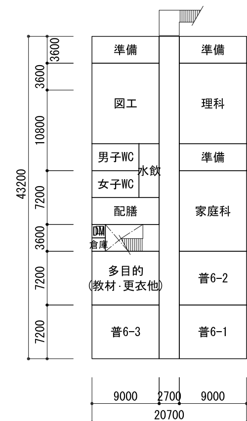
2階 平面図
