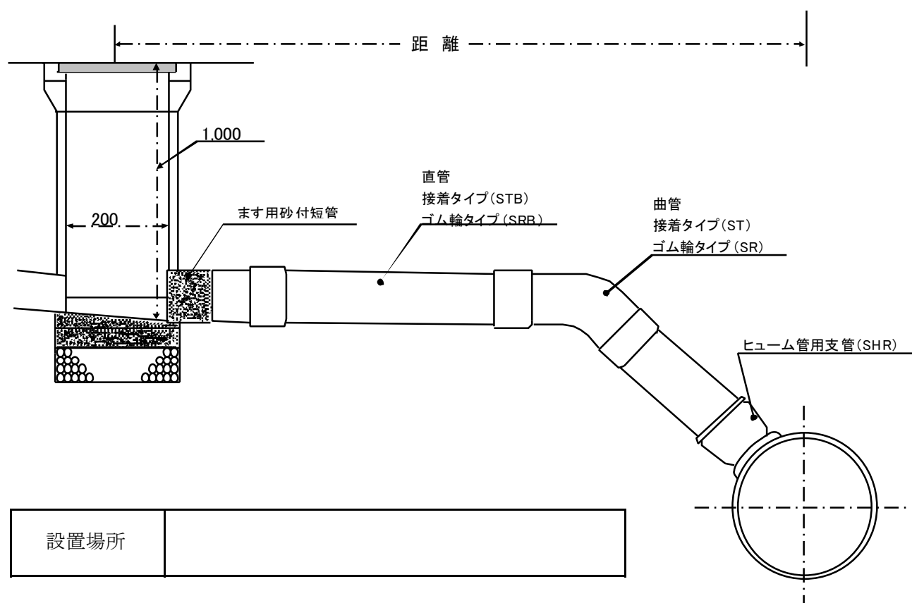
断面図
