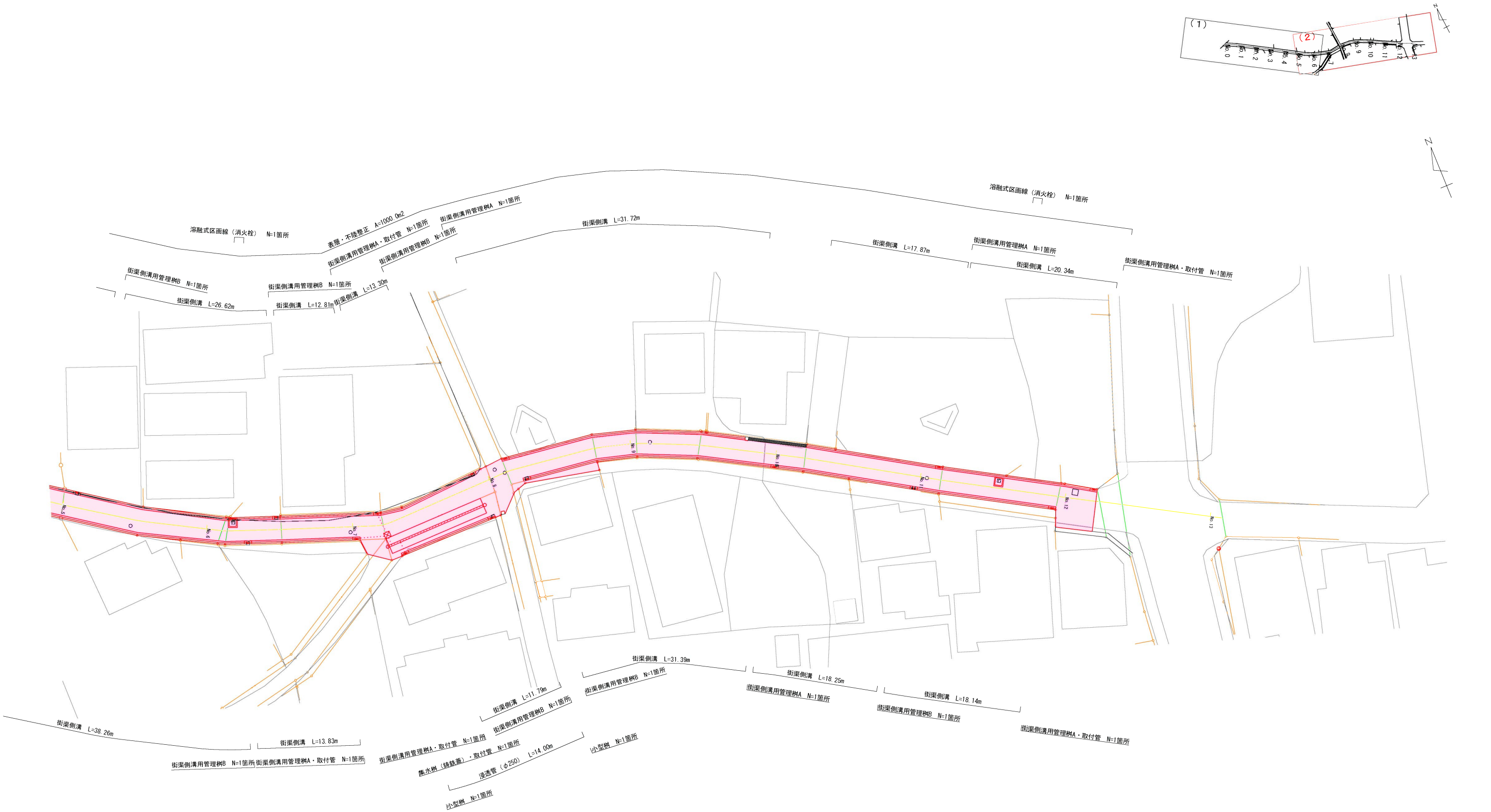
詳細平面図（2） S=1:250
