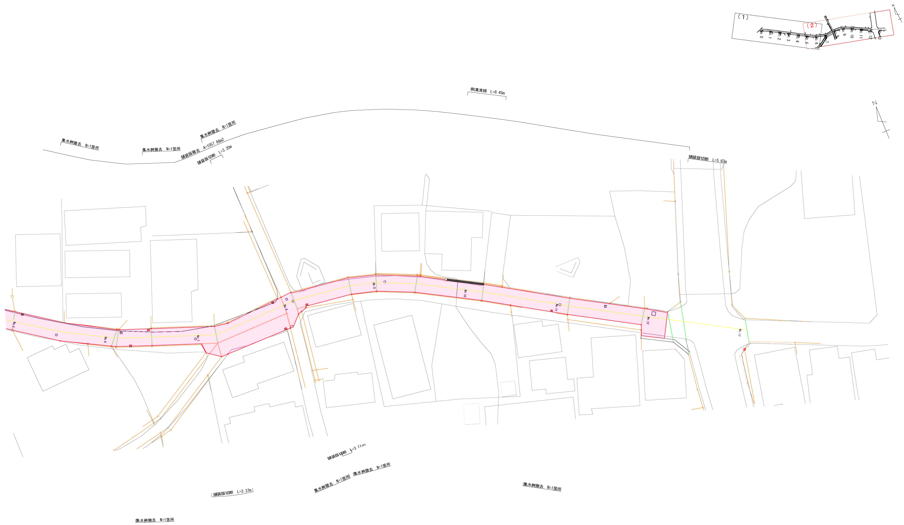
撤去平面図（2） S=1:250
