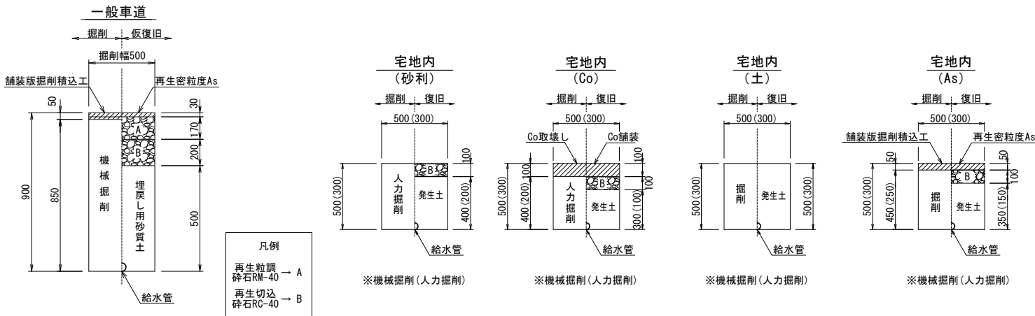
給水土工図 縮尺 Free
