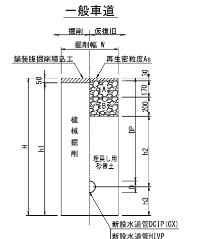
穿孔部土工図 縮尺 1:20
