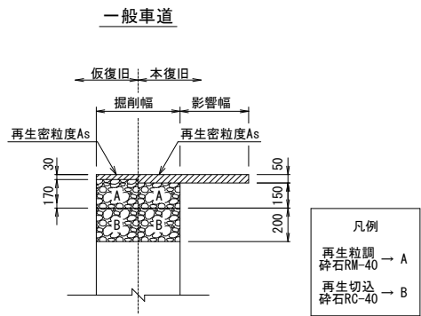
舗装復旧組成図 縮尺 1:20
