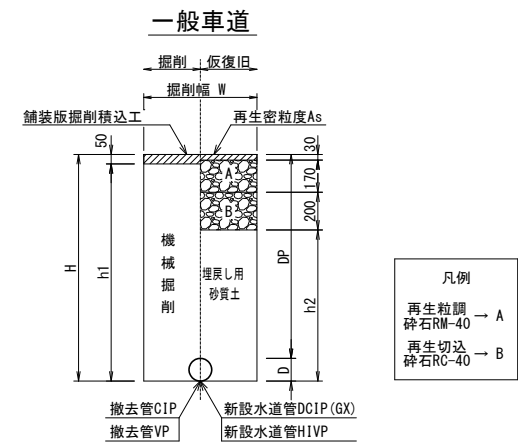
本設土工図 縮尺 1:20
