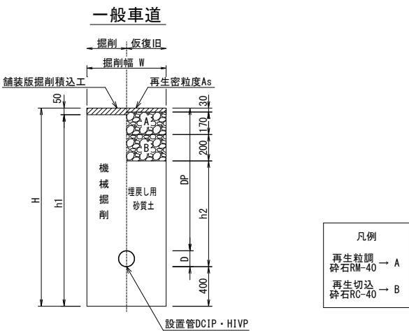
不断水分岐土工図 縮尺 1:20
