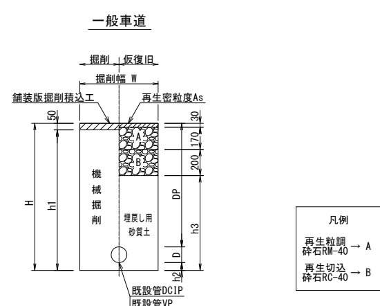
不断水簡易仕切弁土工図 縮尺 1:20
