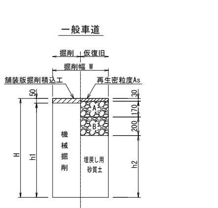
作業用仕切弁土工図 縮尺 1:20
