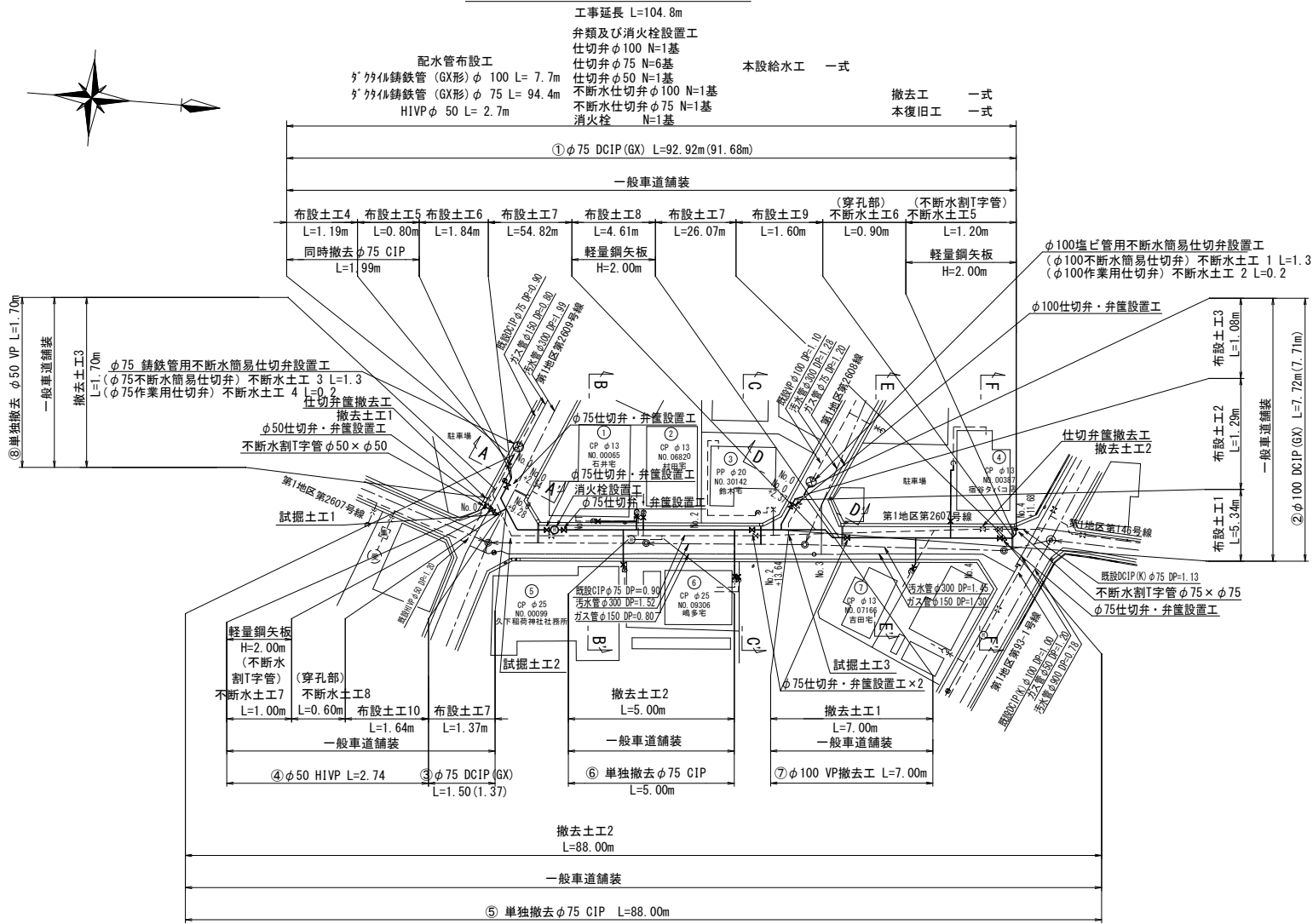
平面図 縮尺 1:500
