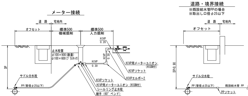
給水詳細図 縮尺 Free
