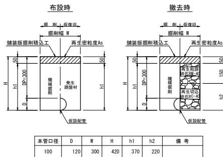
仮設土工図 縮尺 1:20
