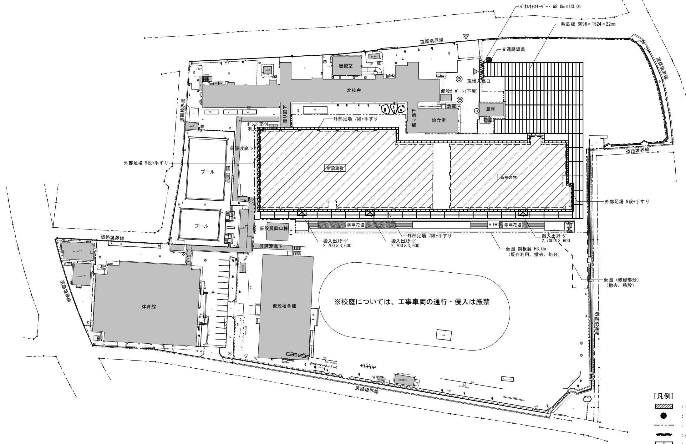
仮設計画図 (参考)
