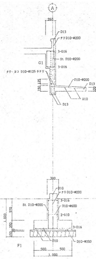
断面配筋図 S=1:30
