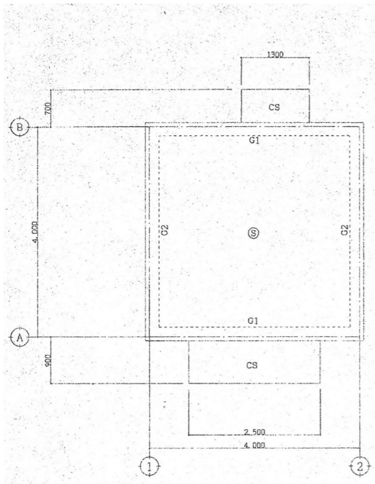
屋根伏図 S=1:50
