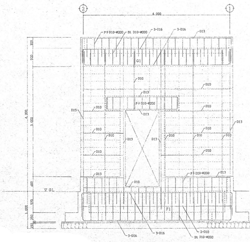
B通り配筋図 S=1:30
