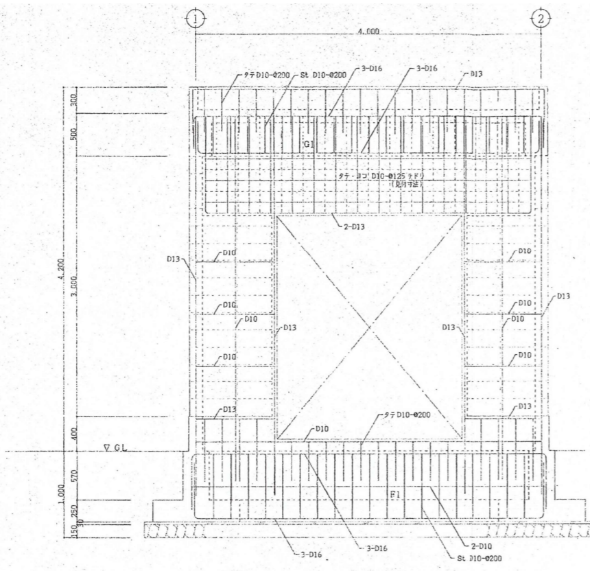
A通り配筋図 S=1:30
