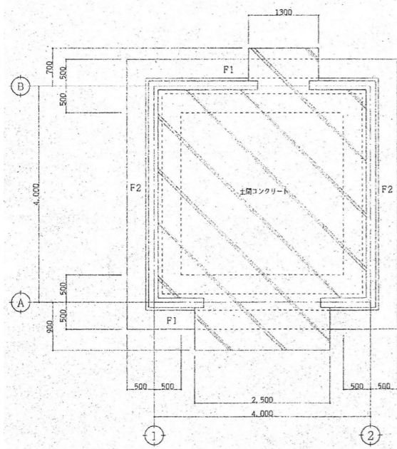
基礎伏図 S=1:50
