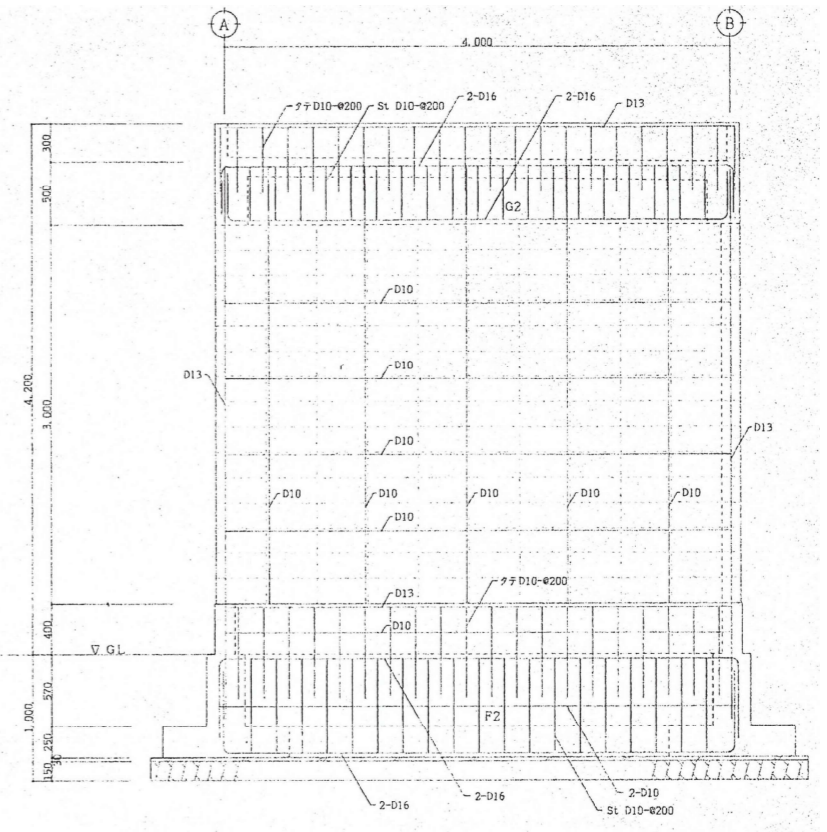
1・2通り配筋図 S=1:30
